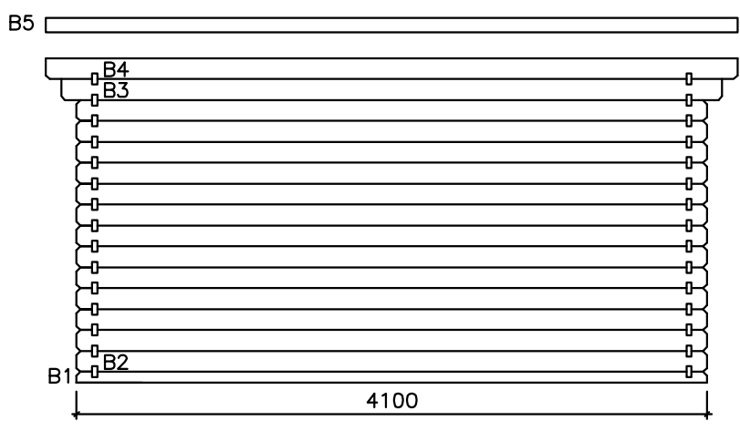
Lillevilla Olos: 3900 x 3000 mm
